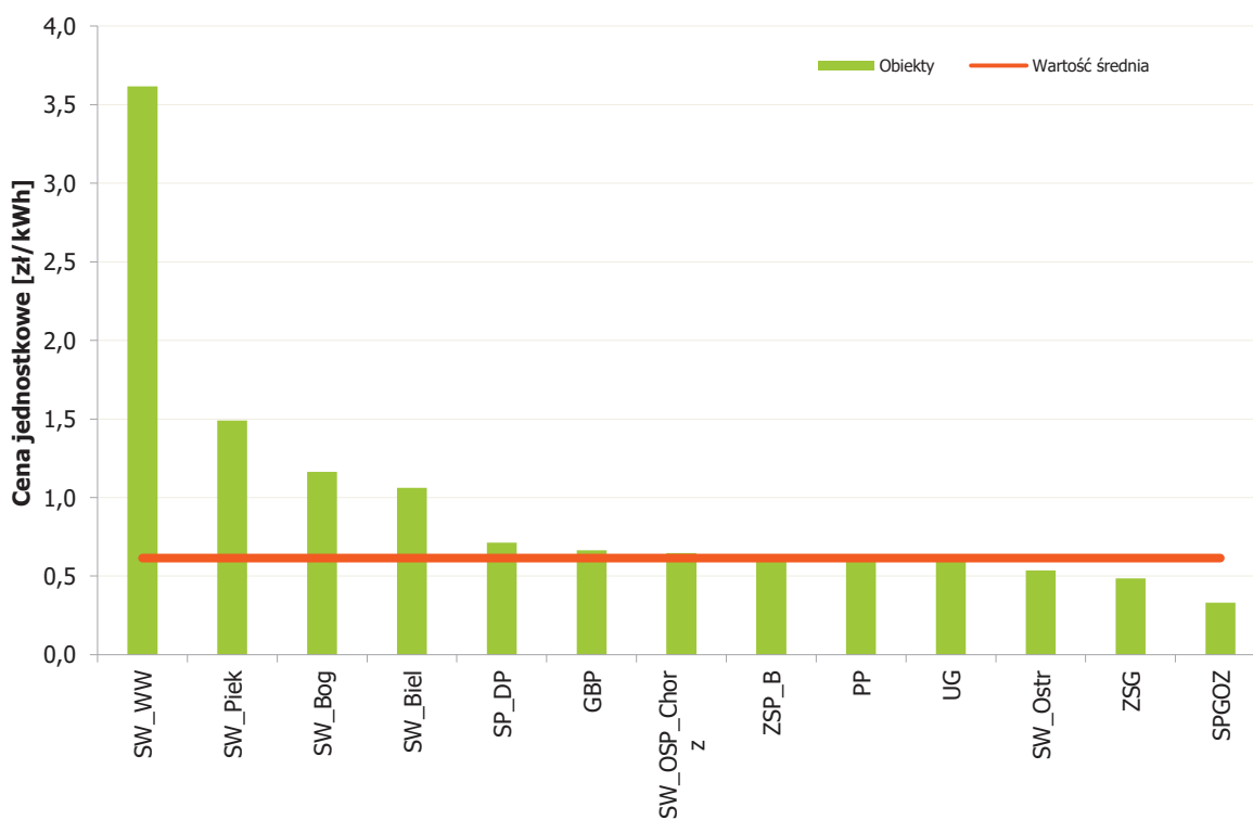
Rysunek 4-5 Porównanie ceny energii elektrycznej dla poszczególnych obiektów
