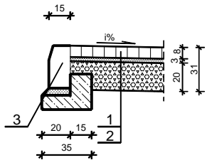
SZCZEGÓŁ "A" 1:20
