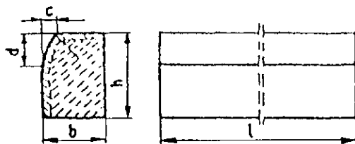
Rys. 1. Wymiarowanie krawężników
