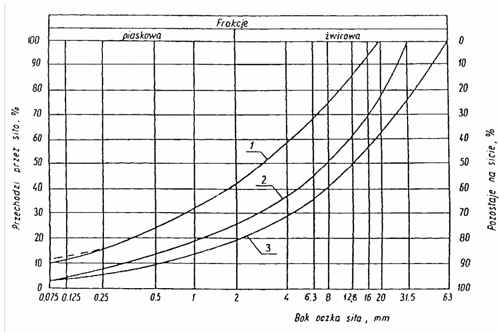
Rysunek 1. Pole dobrego uziarnienia kruszywa przez naczynach na podbudowy wykonanych metodą stabilizacji mechanicznej
