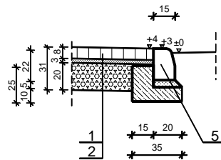
SZCZEGÓŁ "B" 1:20
