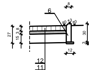
"DOJŚCIE DO KAPLICZKI" 1:20
