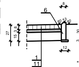
SZCZEGÓŁ "C" 1:20
