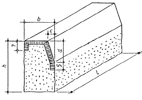
Rys. 1. Krawężnik uliczny odmiany UP, rodzaju A
