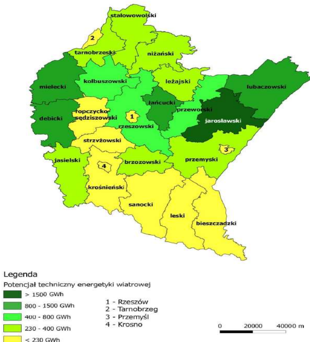
Mapa 7. Potencjał techniczny energetyki wiatrowej w województwie Podkarpackim
