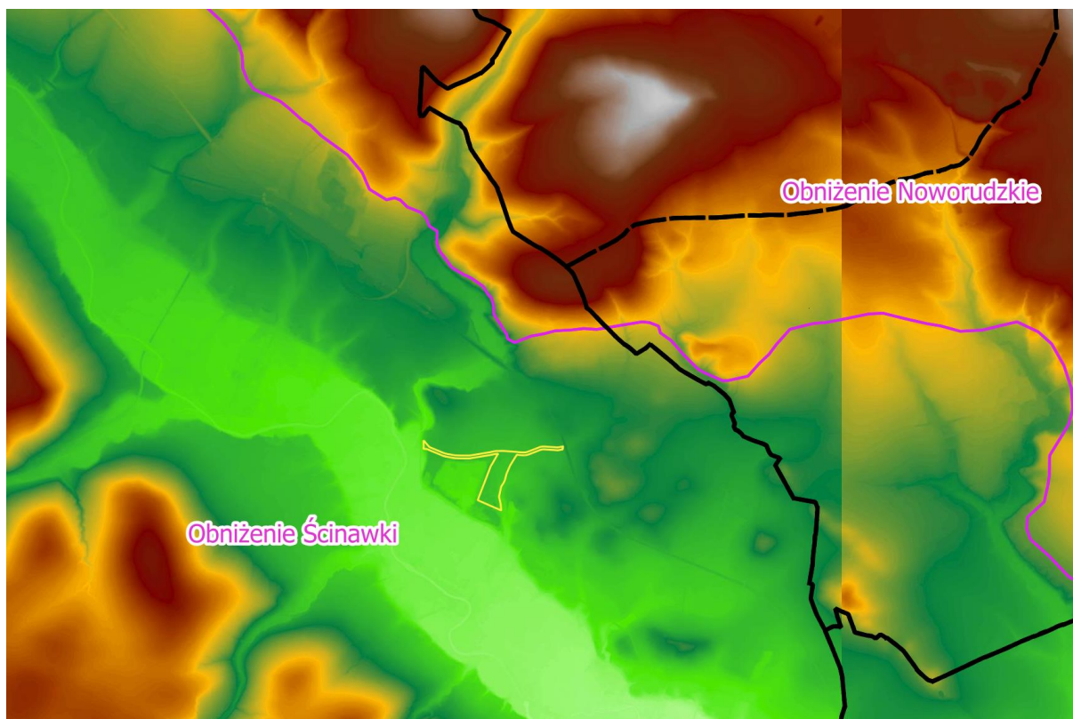
Rysunek 9. Położenie fizyczno - geograficzne obszaru objętego projektem planu
