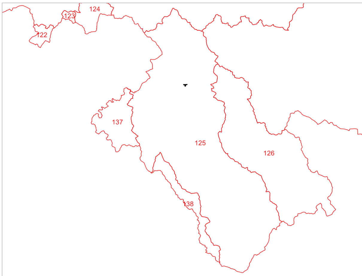
Rysunek 12. Obszar objęty projektem planu w całości położony jest na terenie JCWPd 125 [źródło: Państwowa Służba Hydrogeologiczna]
