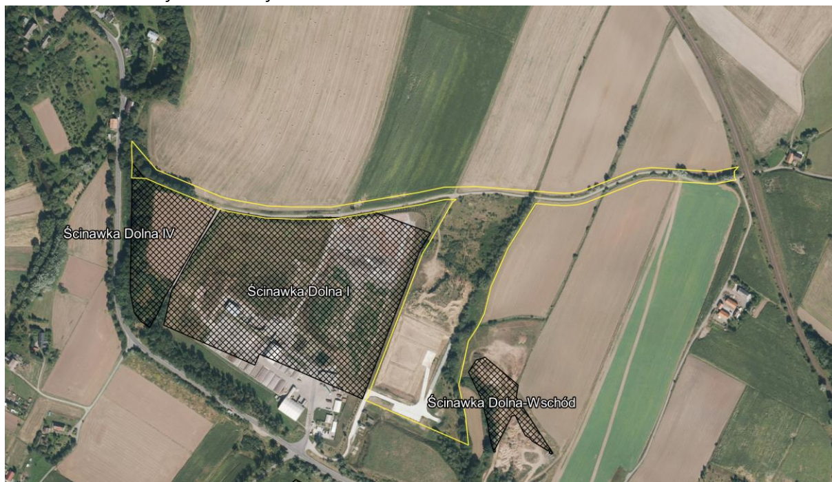
Rysunek 10. Udokumentowane złoża kopalin w sąsiedztwie projektu zmiany planu
