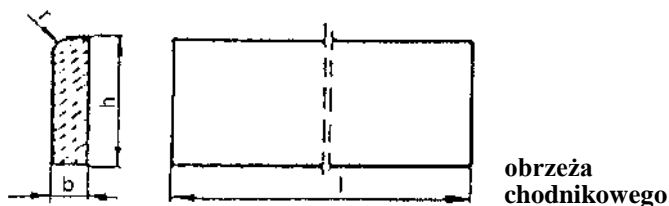
Rysunek 1. Kształt betonowego obrzeża chodnikowego. Tablica 1. Wymiary obrzeży
