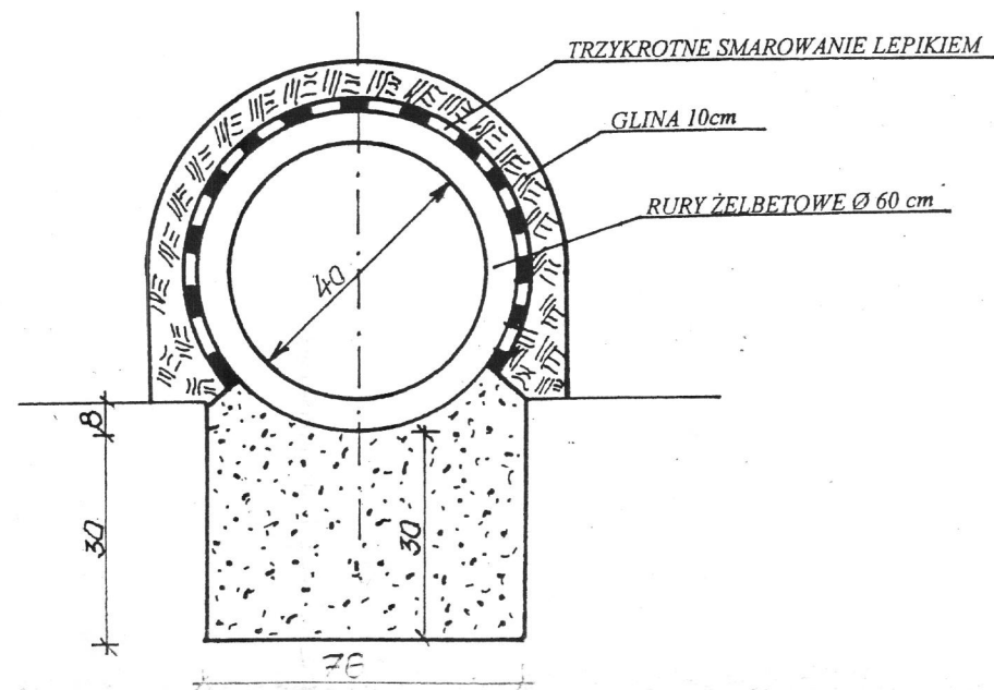
POSADOWIENIE RUR W PRZEPUŚCIE 1:20
