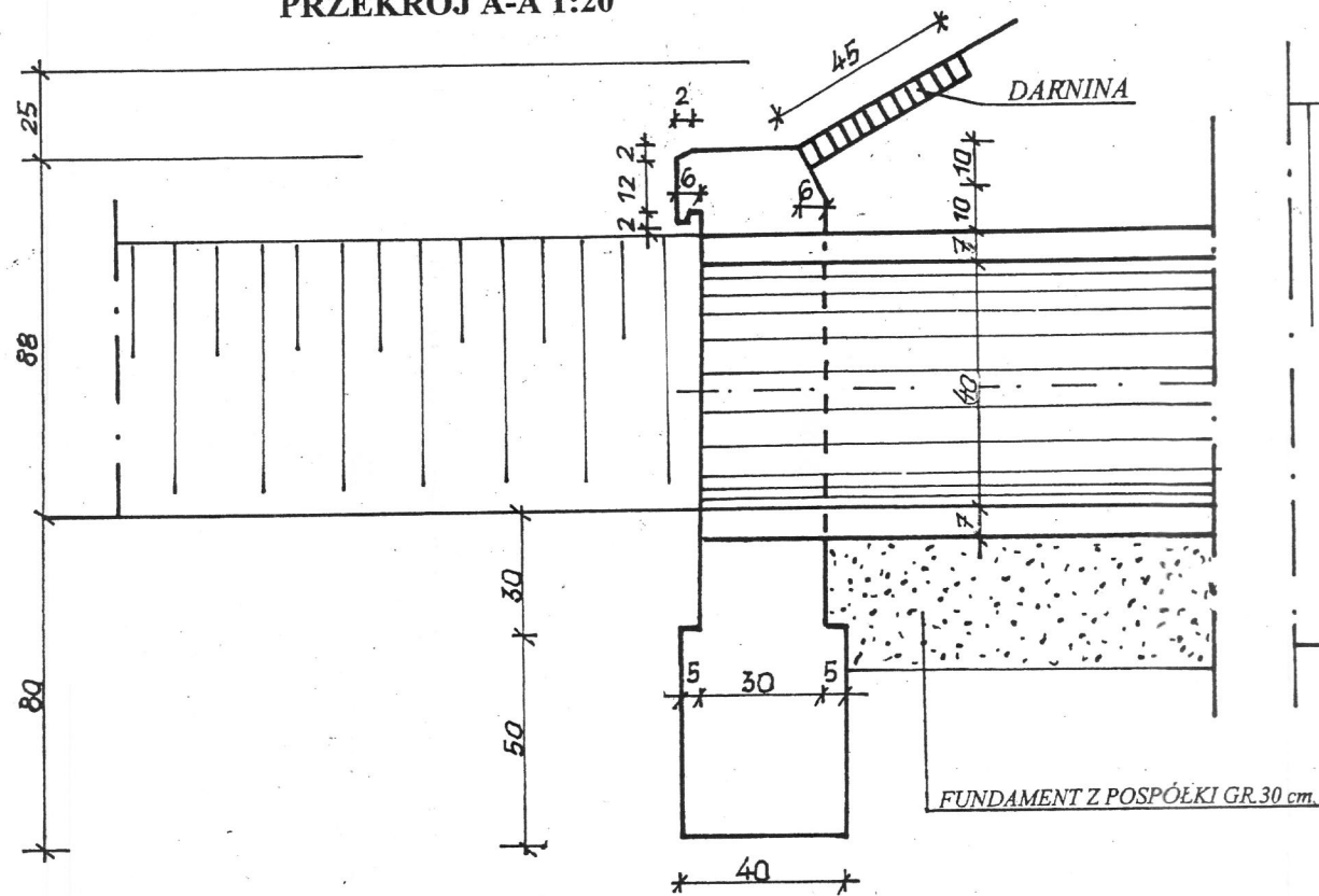
POSADOWIENIE RUR W PRZEPUŚCIE 1:20
