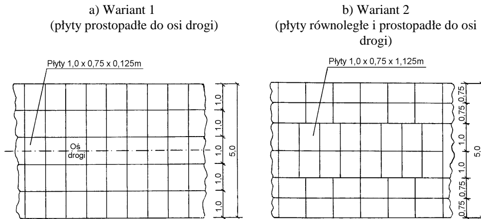
Rys. 3. Przykład ułożenia płyt według systemu płatowego na jezdni dwupasowej szerokości 5 m
