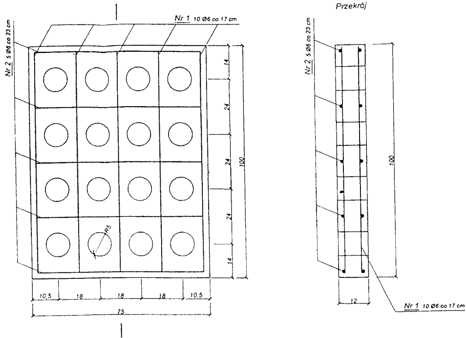
c) Płyta 1,0 \times 0,75 \times 0,125 m z otworami okrągłymi
