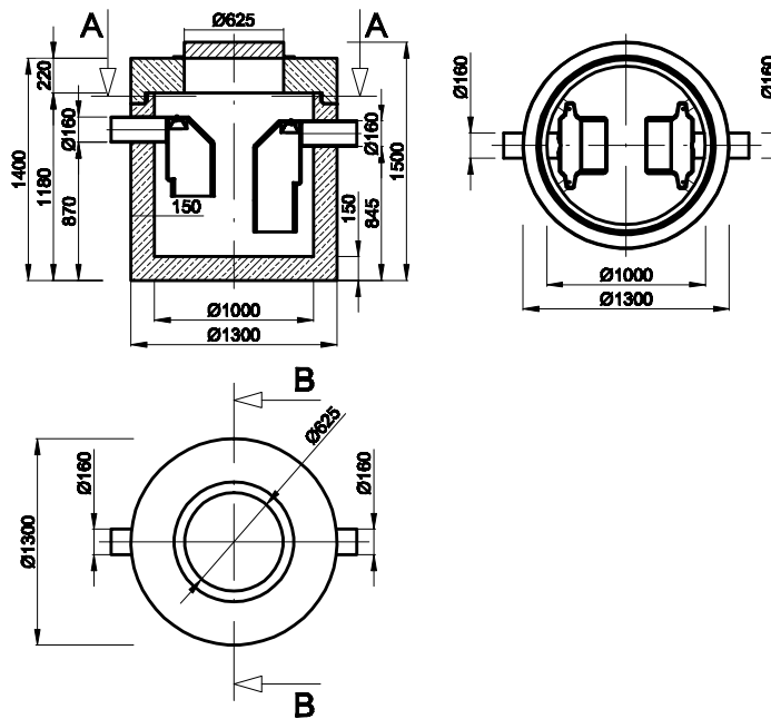
PRZEKRÓJ B:B
