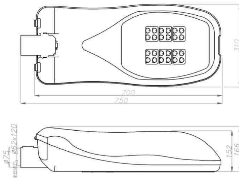
Rysunek nr 2 Wizerunek oprawy
