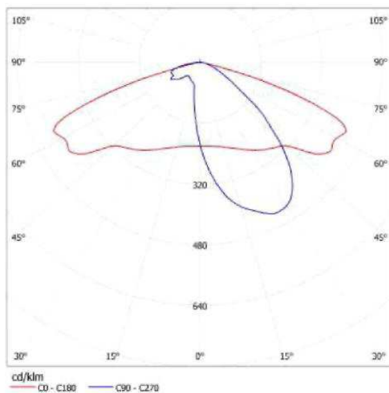
Rysunek nr 1: Krzywa rozsyłu opraw przyjętej w obliczeniach
