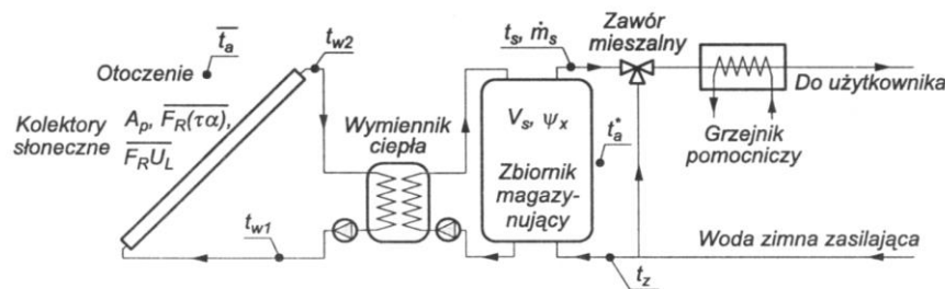
Rys. 86 Standardowa konfiguracja aktywnego systemu przygotowania ciepłej wody użytkowej. Na rysunku naniesiono parametry instalacji będące danymi wejściowymi do metody f - chart przystosowanej do obliczeń słonecznej instalacji cwu
