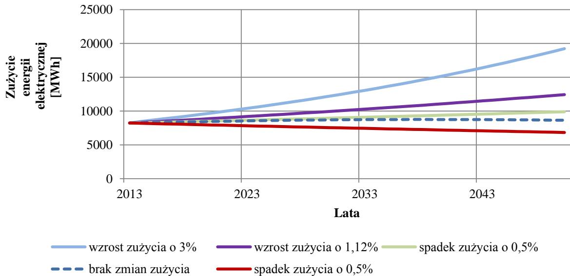
Rys. 19. Prognoza jednostkowego zużycia energii elektrycznej dla Gminy Lipusz do roku 2050
