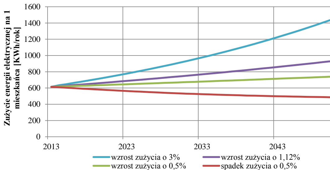
Rys. 17. Progniza jednostkowego zużycia energii elektrycznej dla Gminy Dziemiany do roku 2050 Źródło: Opracowanie własne na podstawie danych GUS
