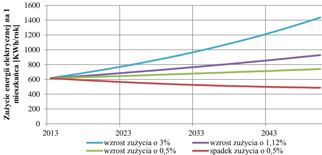
Rys. 7. Prognoza jednostkowego zużycia energii elektrycznej dla Gminy Kościerzyna do roku 2050 Źródło: Opracowanie własne na podstawie danych GUS
