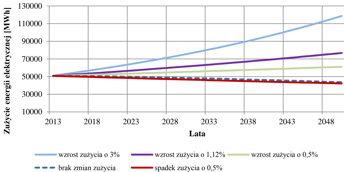
Rys. 3. Progniza całkowitego zużycia energii dla Gminy Miejskiej Kościerzyna do roku 2050 Źródło: opracowanie własne na podstawie danych GUS
