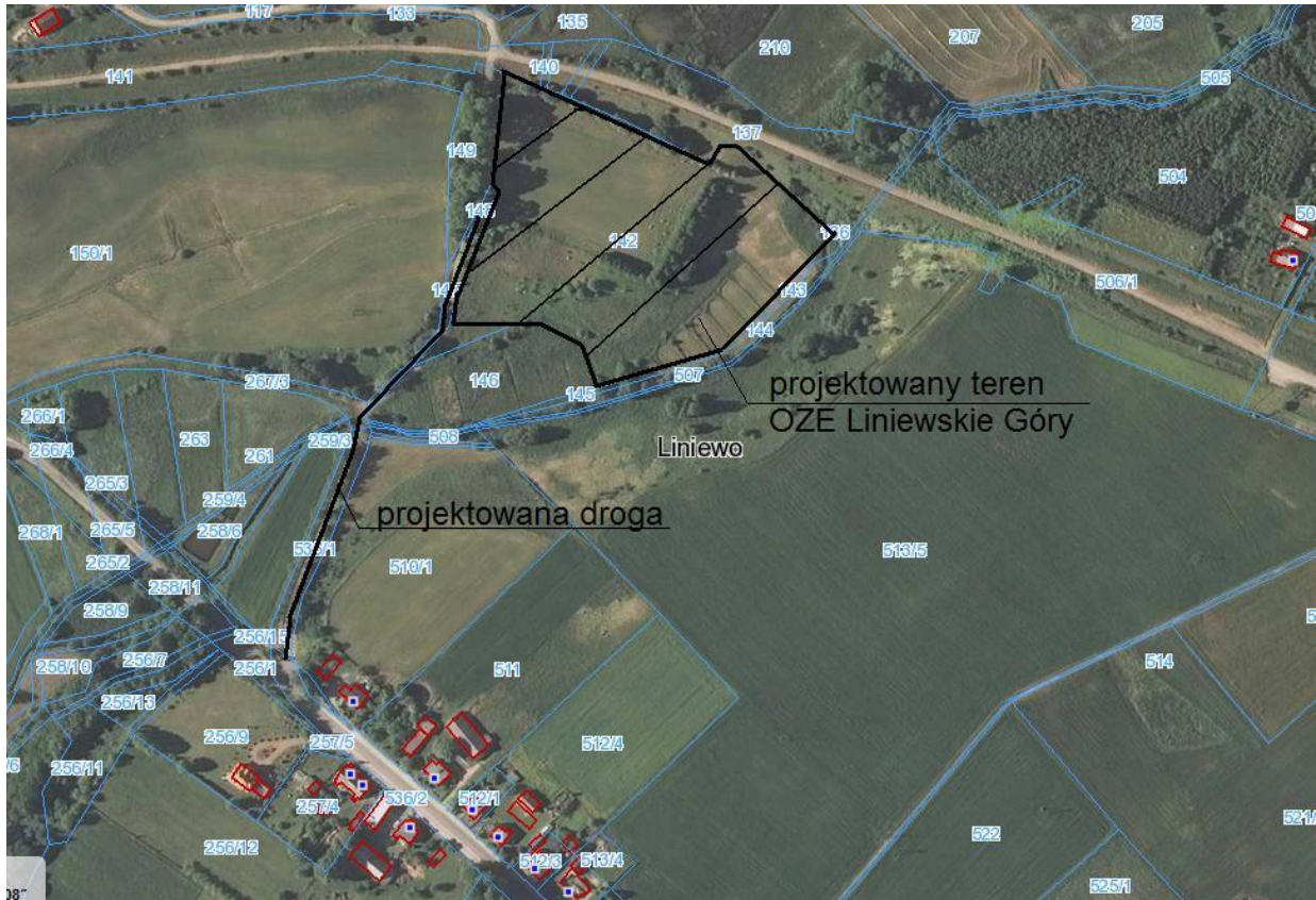
Rys. 93. Projektowany teren OZE Liniewskie Góry
