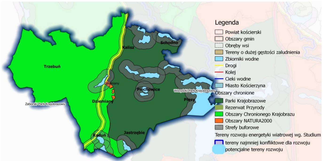
Rys. 71. Potencjalne tereny inwestycyjne pod energetykę wiatrową na terenie gminy Dziemiany Źródło: Opracowanie własne
