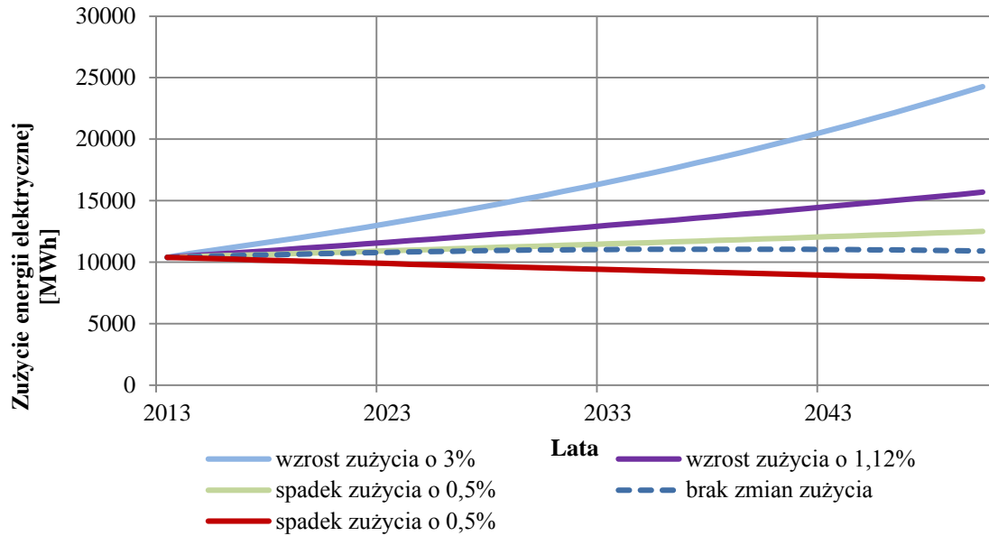
Rys. 16. Progniza całkowitego zużycia energii elektrycznej dla Gminy Dziemiany do roku 2050 Źródło: Opracowanie własne na podstawie danych GUS
