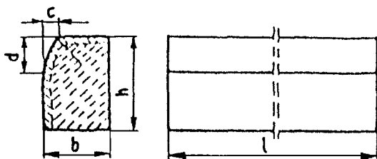
Tablica 2. Dopuszczalne odchyłki wymiarów krawężników betonowych
