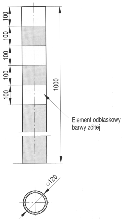
Rys. . Słupek krawędziowy U-2
