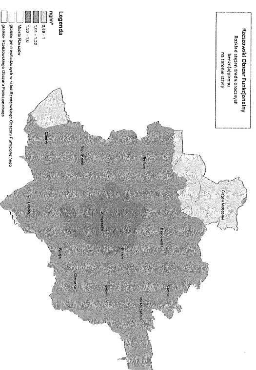
Rysunek 64. Rozkład stężeń średniorocznych benzo(a)pirenu na terenie Rzeszowskiego Obszaru Funkcjonalnego w roku bazowym 2013 275
