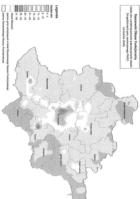
Rysunek 62. Rozkład liczby dni z przekroczeniem dopuszczalnej wartości stężenia 24-godzinnego dla pyłu zawieszonego PM10 w Rzeszowskim Obszarze Funkcjonalnym w roku bazowym 2013 73
