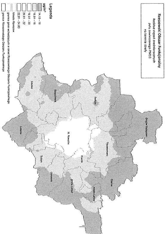
Rysunek 61. Rozkład stężeń średniorocznych pyłu zawieszonego PM10 w Rzeszowskim Obszarze Funkcjonalnym w roku bazowym 2013 72
