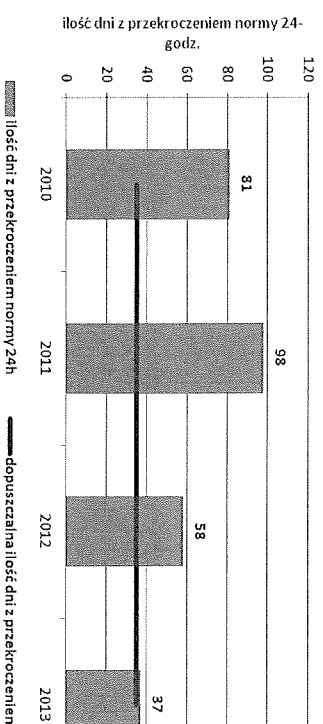
Rysunek 6. Liczba dni z przekroczeniem normy 24 -godz. pyłu zawieszzonego PM10 na przetrzeni lat 2010-2013, na stacji pomiarowej Rzeszów – ul. Szopena i Rzeszów – osiedle Nowe Miasto 42
