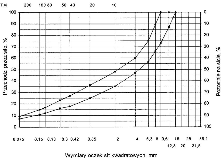
Rys. 7. Krzywe graniczne uziarnienia mieszanki mineralnej BA od 0 do 12,8 mm do warstwy ścierylnej nawierzchni drogi o obciążeniu ruchem od KR3 do KR6
