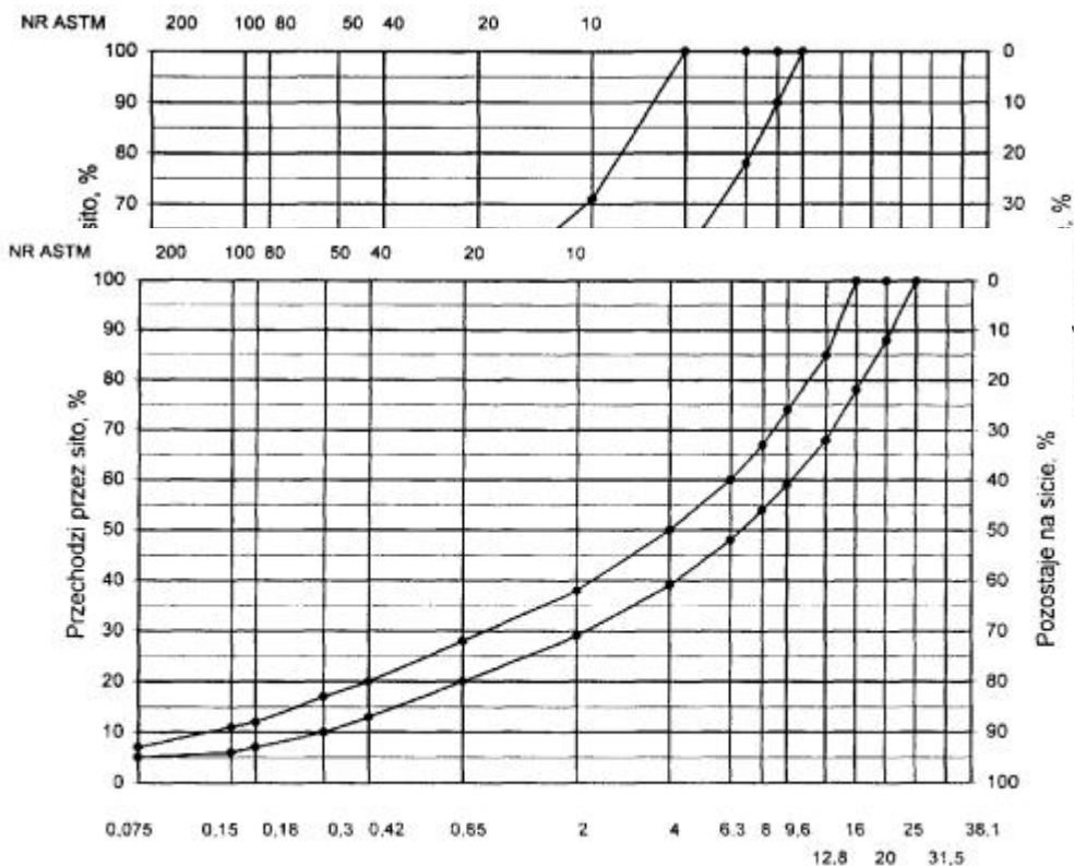
Rys. 3. Krzywe graniczne uziarnienia mieszanki mineralnej BA od 0 do 8mm, od 0 do 6,3 mm do warstwy ścieralnej nawierzchni drogi o obciążeniu ruchem nawierzchni drogi o obciążeniu ruchem KR1 lub KR2
