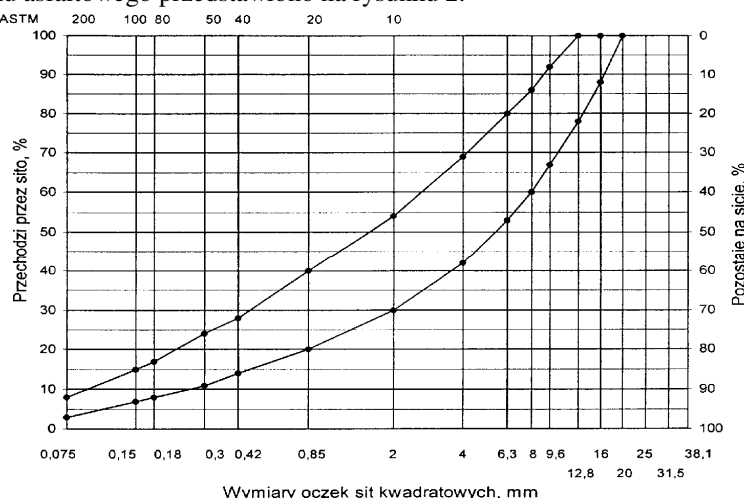
Rys. 2. Krzywe graniczne uziarnienia mieszanki mineralnej BA od 0 do 16 mm do warstwy wiążącej, wyrównawczej i wzmacniającej nawierzchni drogi o obciążeniu ruchem KR1 lub KR2
