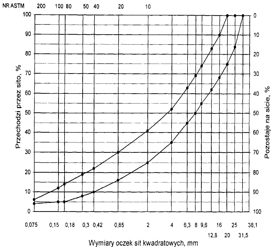
Rys. 12. Krzywe graniczne uziarnienia mieszanki mineralnej BA od 0 do 20 mm do warstwy wiążącej, wyrównawczej i wzmacniającej nawierzchni drogi o obciążeniu ruchem od KR3 do KR
