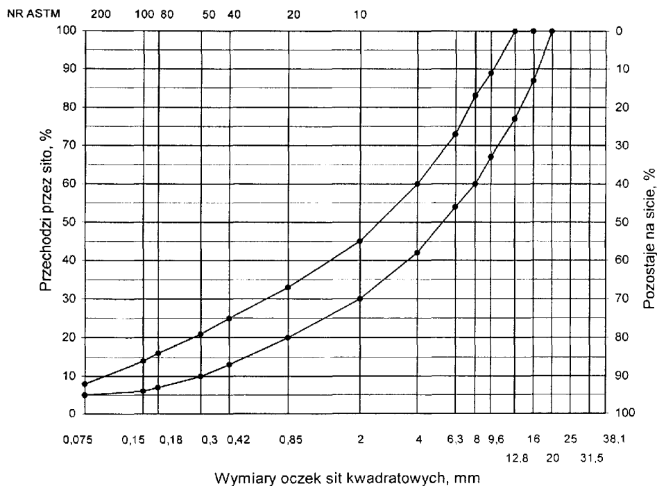
Rys. 12. Krzywe graniczne uziarnienia mieszanki mineralnej BA od 0 do 20 mm do warstwy wiążącej, wyrównawczej i wzmacniającej nawierzchni drogi o obciążeniu ruchem od KR3 do KR
