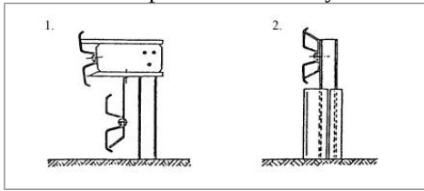
1 - dodatkowa prowadnica bariery
