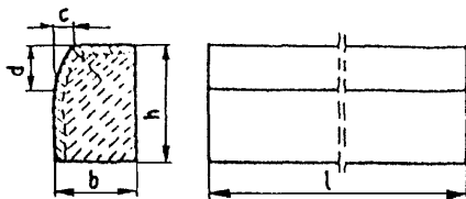
Rys. 1. Wymiarowanie krawężników
