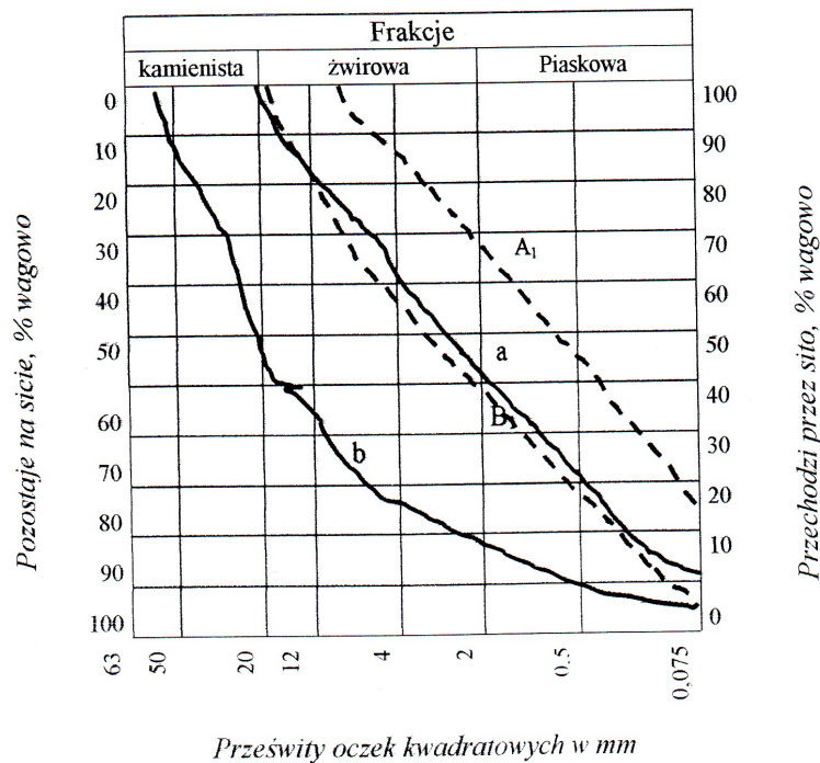
Rysunek 1. Obszar uziarnienia optymalnych mieszanek żwirowych
