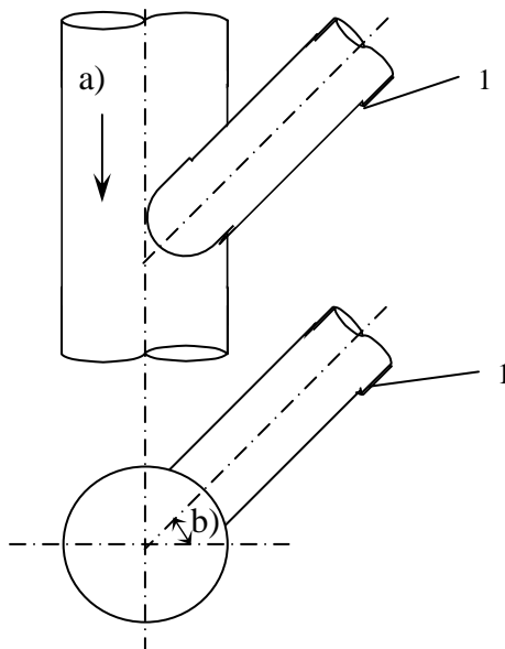
Rys. 2: Odgałęzienie
