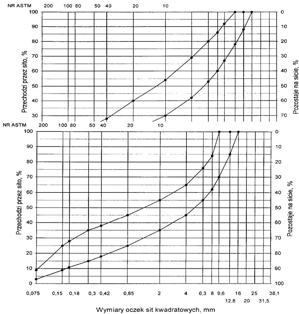
Rys. 10. Krzywe graniczne uziarnienia mieszanki mineralnej BA od 0 do 12,8 mm do warstwy wiążącej, wyrównawczej i wzmacniającej nawierzchni drogi o obciążeniu ruchem KR1 lub KR2
