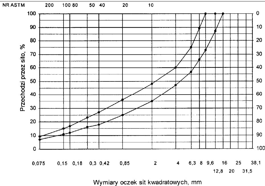
Rys. 7. Krzywe graniczne uziarnienia mieszanki mineralnej BA od 0 do 12,8 mm do warstwy ścieralnej nawierzchni drogi o obciążeniu ruchem od KR3 do KR6 Skład mieszanki mineralno-asfaltowej powinien być ustalony na podstawie badań próbek wykonanych wg metody Marshalla. Próbkę powinny spełniać
