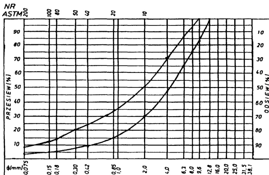
Rys. 2. Krzywe graniczne uziarnienia mieszanki mineralnej 0÷12,8 mm do podbudowy z betonu asfaltowego dla KR 1-2.
