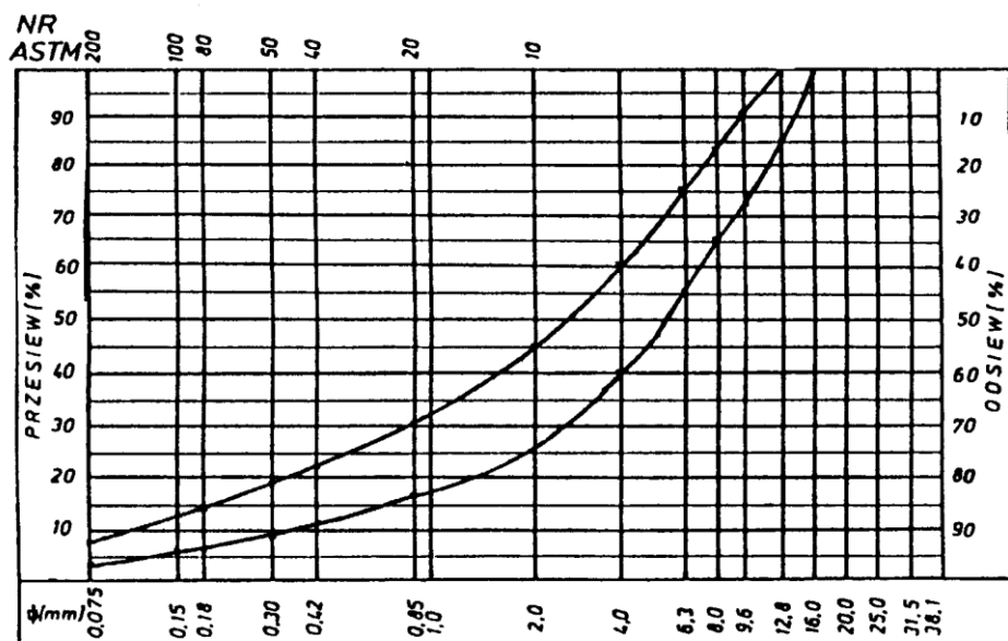
Rys. 1. Krzywe graniczne uziarnienia mieszanki mineralnej 0÷16 mm do podbudowy z betonu asfaltowego dla KR 1-2
