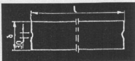
Rys. 1. Wymiarowanie krawężników
