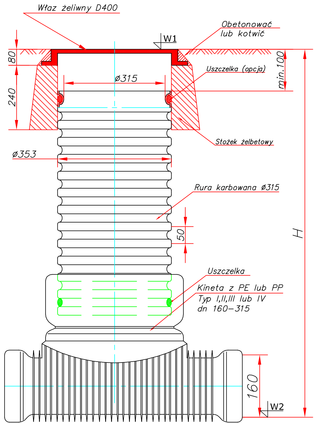
Studzienka inspekcyjna Ø315 na sieci
