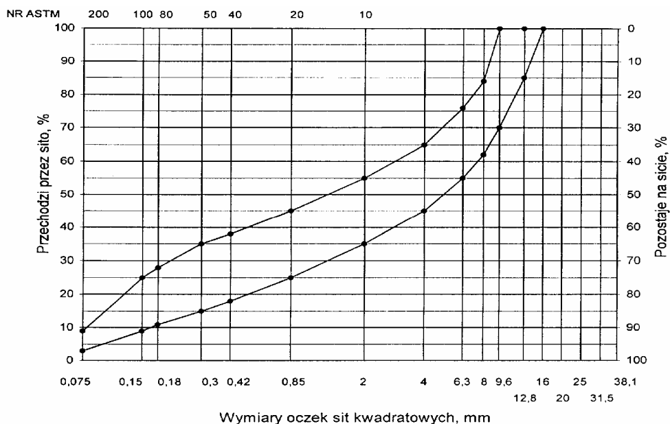
Rys. 10. Krzywe graniczne uziarnienia mieszanki mineralnej BA od 0 do 12,8 mm do warstwy wiążącej nawierzchni drogi o obciążeniu ruchem KR1 lub KR2
