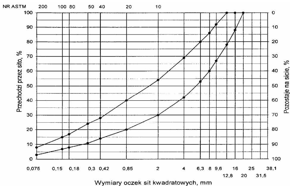
Rys. 9. Krzywe graniczne uziarnienia mieszanek mineralnej BA od 0 do 16 mm do warstwy wiążącej nawierzchni drogi o obciążeniu ruchem KR1 lub KR2
