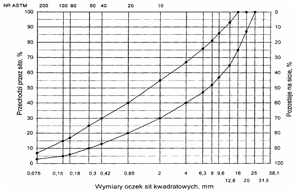
Rys. 8. Krzywe graniczne uziarnienia mieszanek mineralnej BA od 0 do 20 mm do warstwy wiążącej nawierzchni drogi o obciążeniu ruchem KR1 lub KR2
