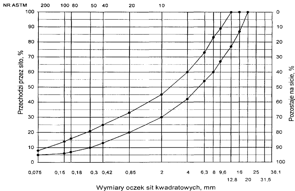
warstwy wyrównawczej nawierzchni drogi o obciążeniu ruchem od KR3 do KR6
