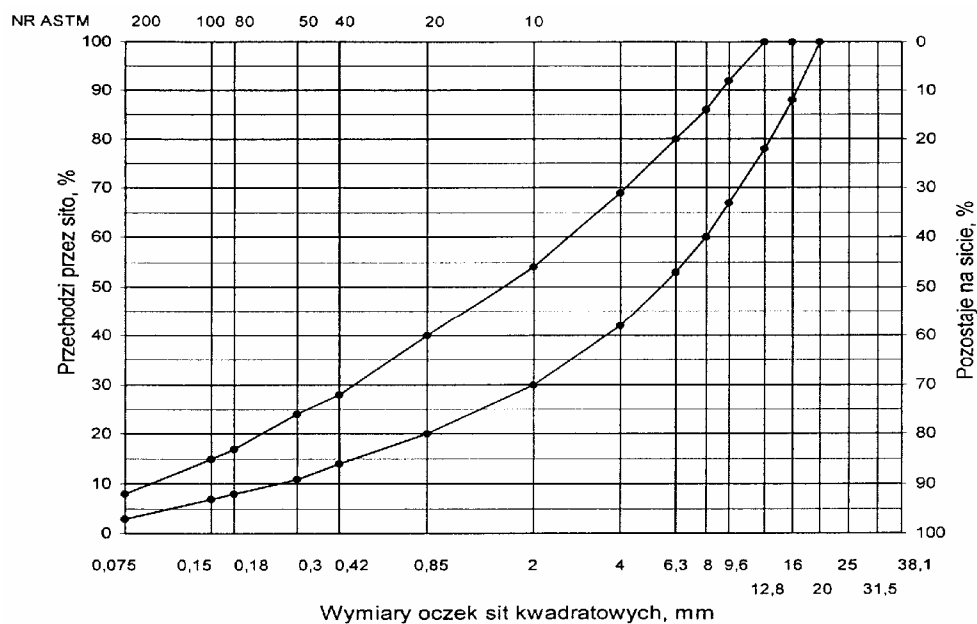
Rys. 9. Krzywe graniczne uziarnienia mieszanki mineralnej BA od 0 do 16 mm do warstwy wiążącej nawierzchni drogi o obciążeniu ruchem KR1 lub KR2
