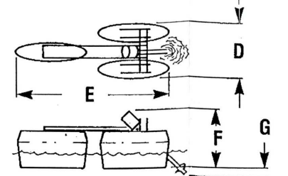
SPOSÓB UMIESZCZENIA ASPIRATORA NA PŁYWAKACH-WIDOK OGÓLNY BEZ SKALI
