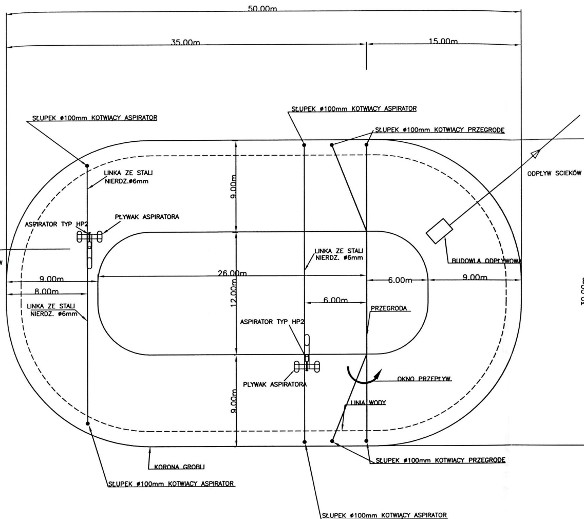
SZCZEGÓŁY ASPIRATORA (WERSJA 50 Hz)
